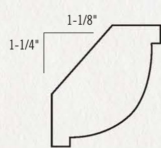
KB321 3/4" x 1-11/16"
