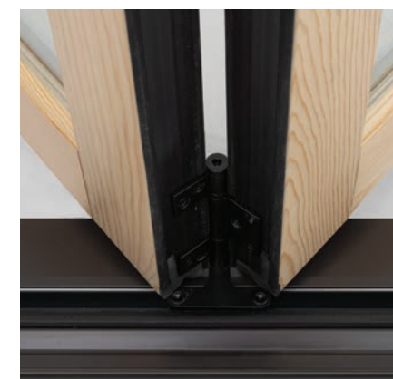
BOTTOM HINGE
