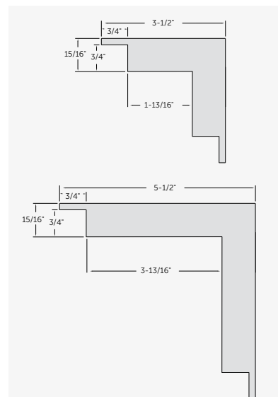
Kleer Konceal® Corner
