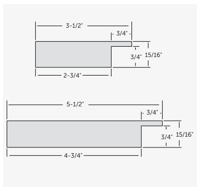
Kleer Konceal® Trimboard
