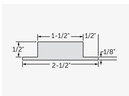
KLEERLok® Moulding
