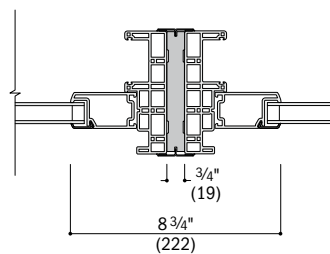
Patio Door Sidelight to Patio Door Sidelight
